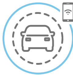
Fahrzeugstatus- Analyse
