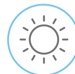
Prévisions météo
